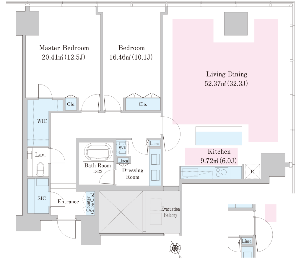
24~29階部分図
